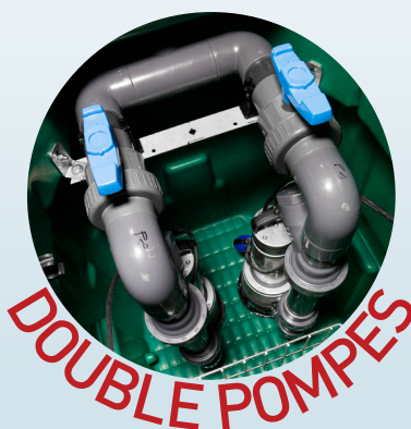
Panier de dégrillage en option
